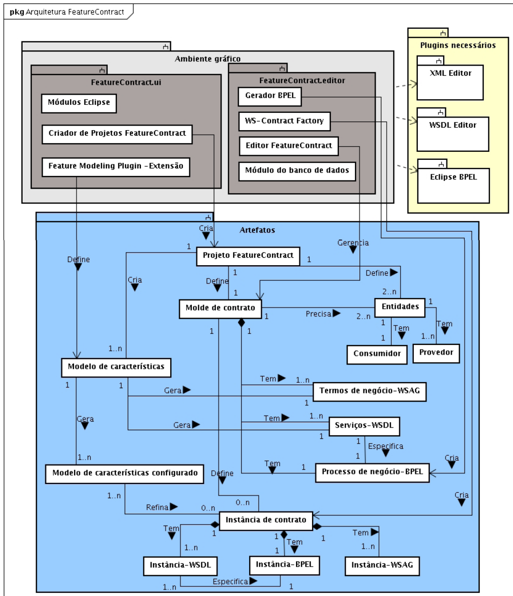
Figura 2 – Arquitetura da ferramenta FeatureContract, em Diagrama de Classes da UML.
